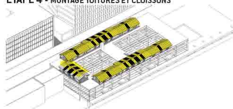
ÉTAPE 4 - MONTAGE TOITURES ET CLOISSONS
